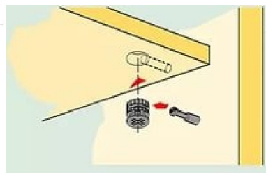
Схема установки Эксцентриковой стяжки
