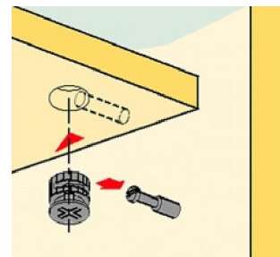
Схема установки Эксцентриковой стяжки
