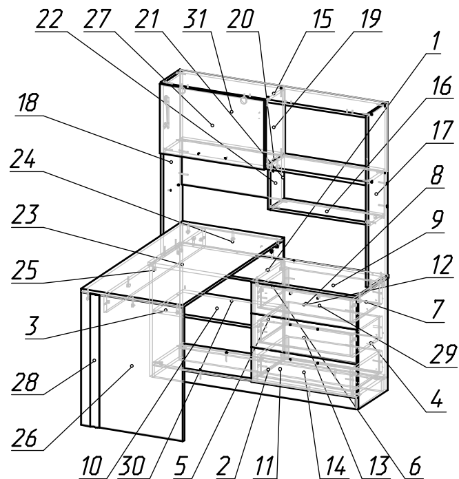
Рис.1 Схема сборки
