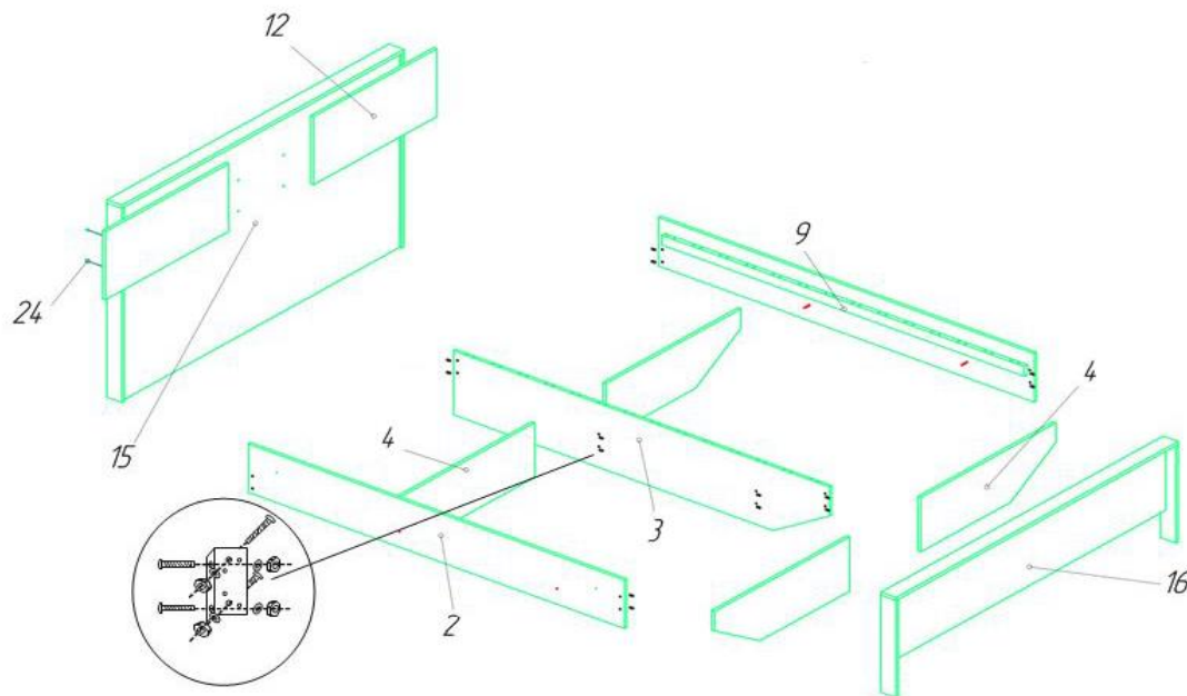
Рисунок 2 – Сборка корпуса кровати
