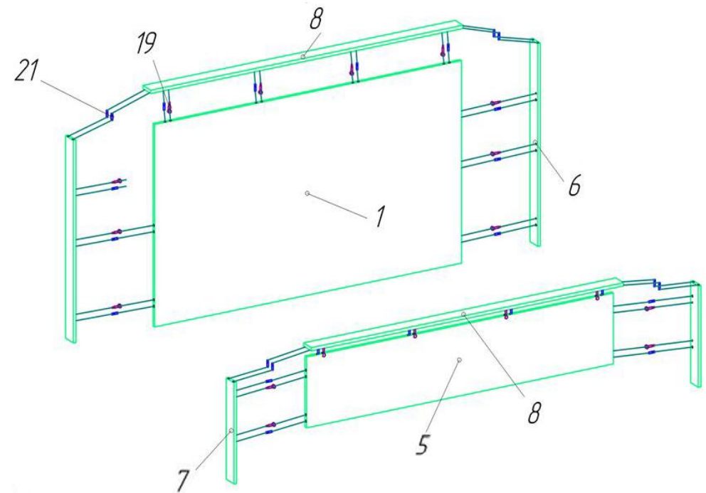
Рисунок 1 – Сборка щитов
