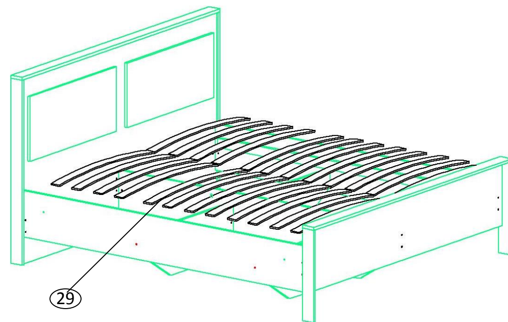
Рисунок 3 – Установка лат
